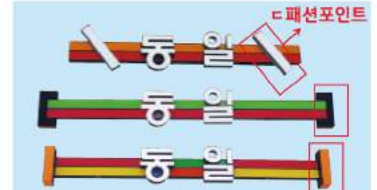
c포인트+200mmAL멀티바+채널바+광학산PC판+시트+AL캡채널+LED+마구리
