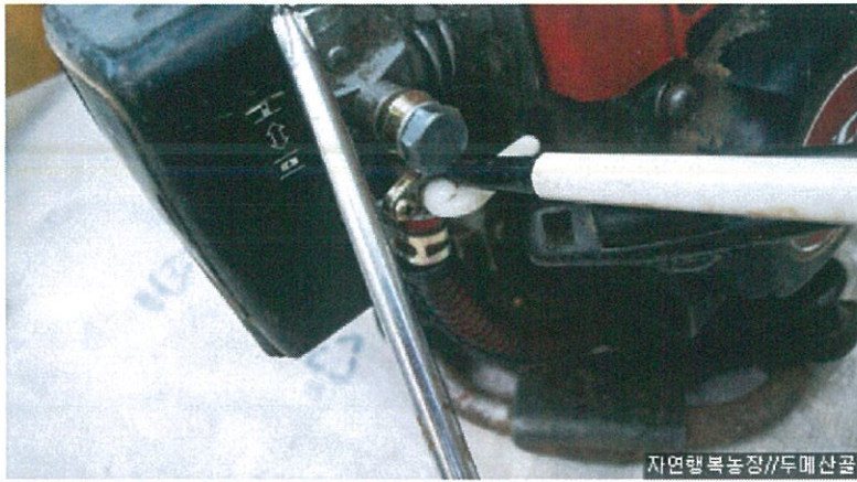
드라이버와 볼펜으로 가리키는 연료 호스는 풀지 말것(연료호스는 잠긴 상태)
